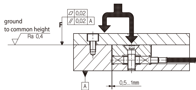
图8：利用9410A型预紧盘组装
