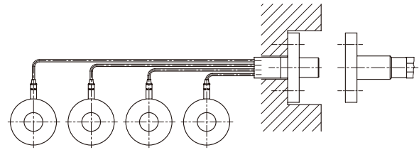
图12: SLS总成
