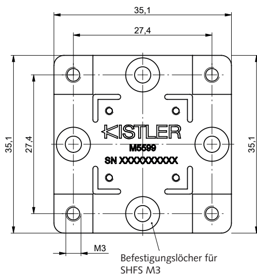
Bild 3: Abmessungen
