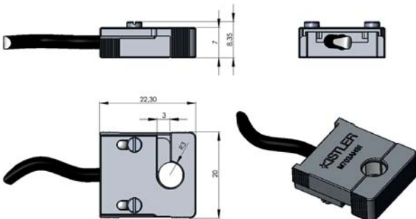
Fig. 3: Dimensions
