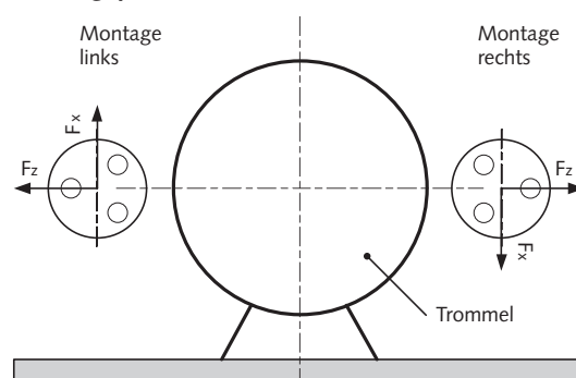
Bild 2: Schema der Messdosensposition am Reifenprüfstand
