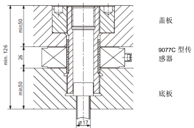
图 4: 通过标准预紧, 安装传感器
