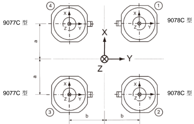
图 3: 四个配套的三分量力传感器组成的 9076C4 型传感器组
