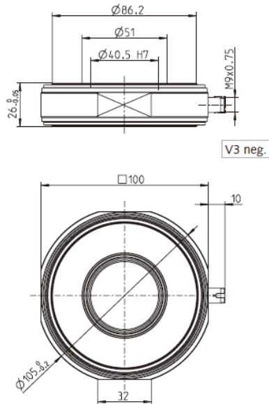
图 1: 9077C 型和 9078C 型外形尺寸
