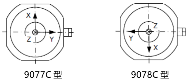
图 2: 9077C 型和 9078C 型三分量力传感器
