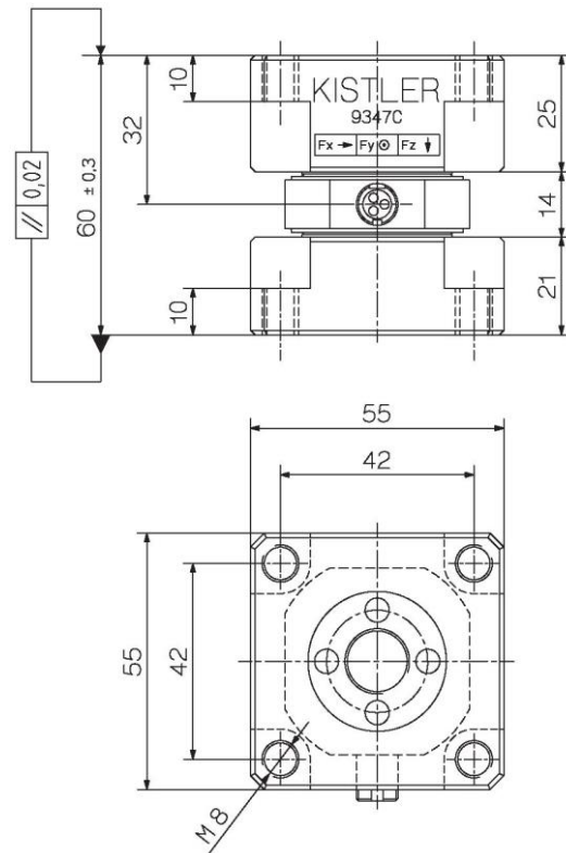
图 2: 9347C 型三分量测力链尺寸
