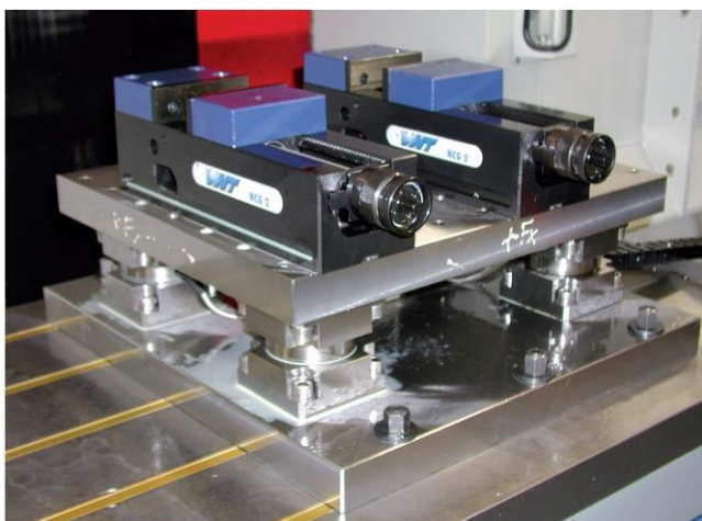
图 1: 由 4 个三分量测力链组成的切削力测力计
