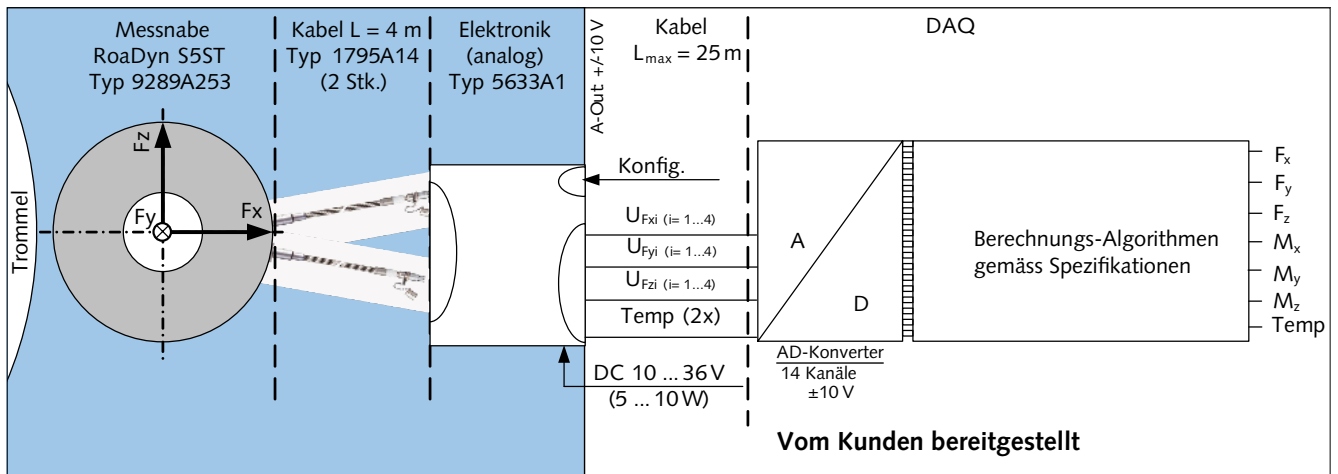
Bild 2: Analoge Messkette RoaDyn® S5ST
