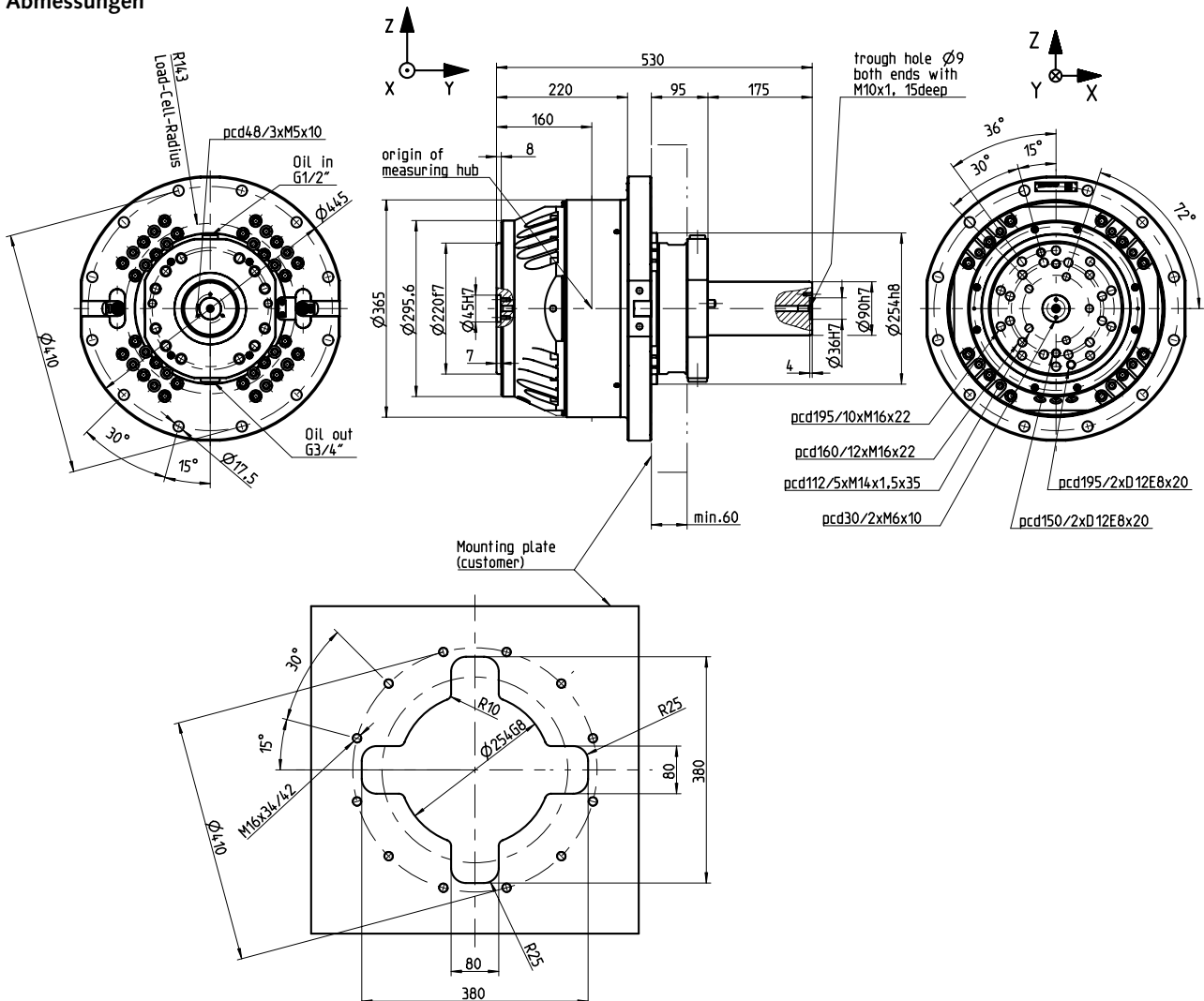
Bild 1: Übersichtszeichnung RoaDyn® S5ST
