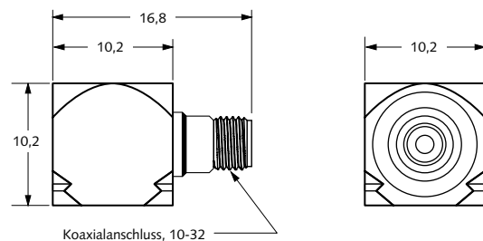
Koaxialanschluss, 10-32
