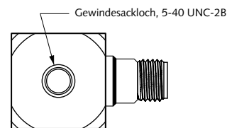
Gewindesackloch, 5-40 UNC-2B
