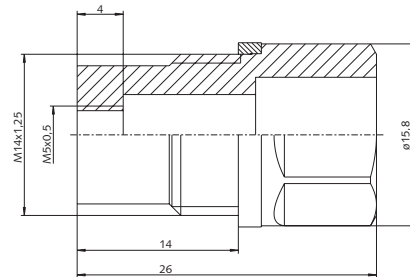
Bild 5: Adapter Typ 6596
