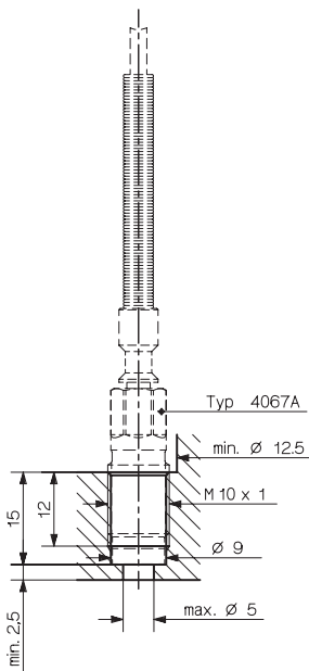
Bild 4: Bohrung für Direktmontage
