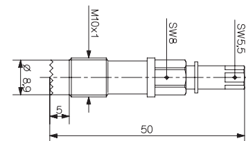
Bild 14: Reibwerkzeug Typ 1300A25
