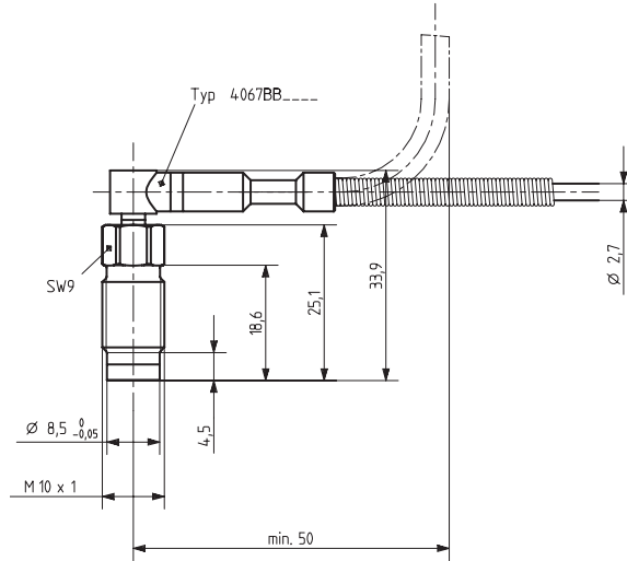
Bild 2: Typ 4067BB...
