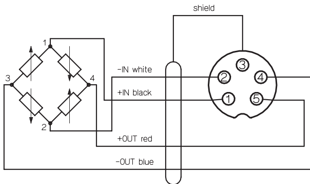
Bild 8: Steckerbelegung Sensor
