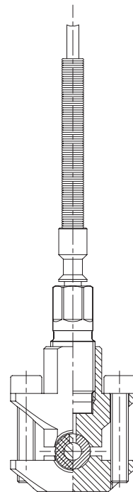
Bild 6: Montage im Bridenadapter Typ 6533A...
