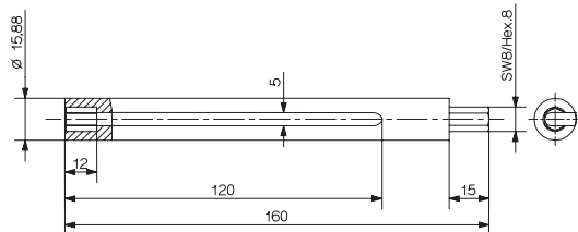
Bild 10: Montageschlüssel für tiefe Bohrungen Typ 1300A41
