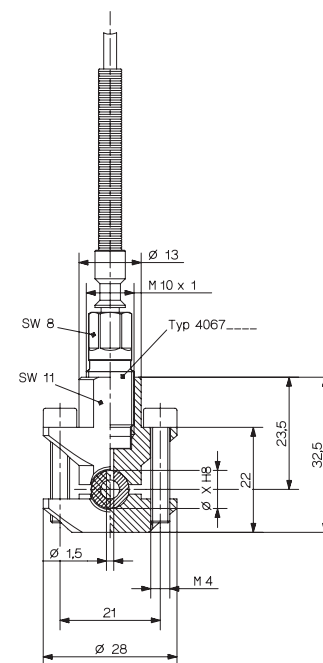
Bild 16: Bridenadapter Typ 6533A1...
