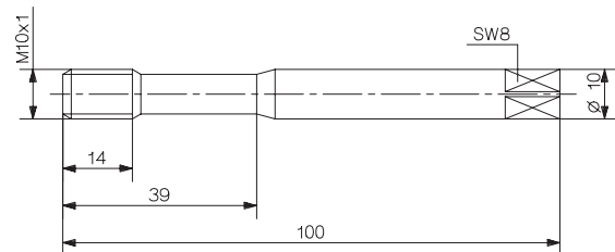
Bild 13: Gewindebohrer Typ 1353
