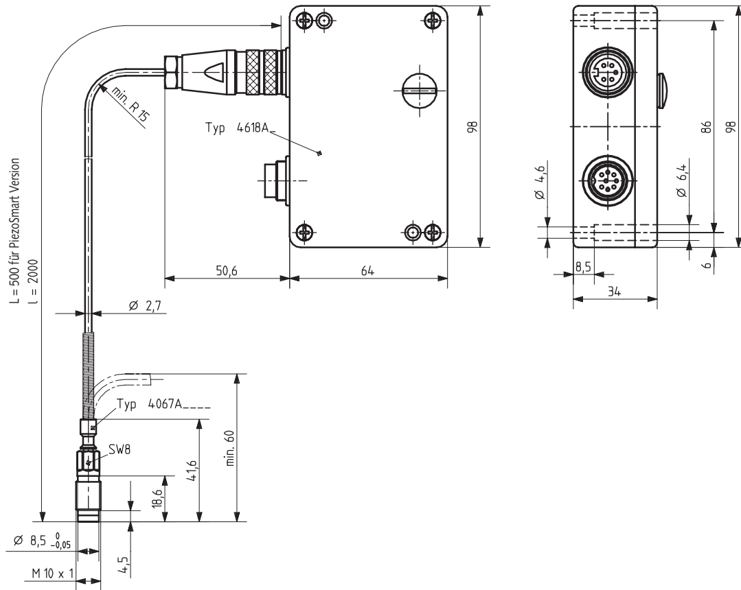
Bild 7: Abmessungen der Messkette
