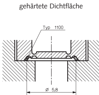
Bild 5: Abdichtung mit Metalldichtung Typ 1100
