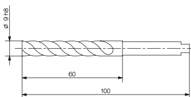
Bild 12: Bohrer Typ 1327
